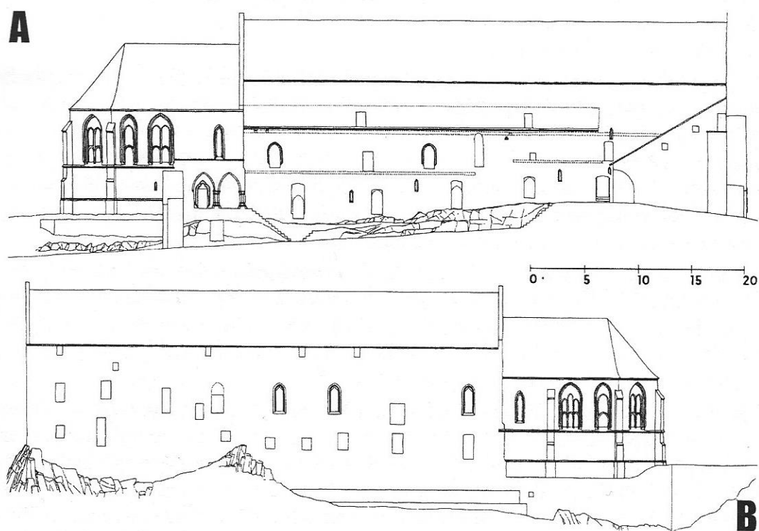
Obr. 3. Bezděz. Průčelí tzv. Královského paláce a kaple. Převzato od D. Menclové (1972, 228, 229). A–hlavní průčelí, B–zadní průčelí. – Abb. 3. Bezděz. Fassade des sog. Königlichen Palas und der Kapelle. Übernommen von D. Menclová (1972, 228, 229). A–Hauptfassade, B–Fassade der Rückseite..
