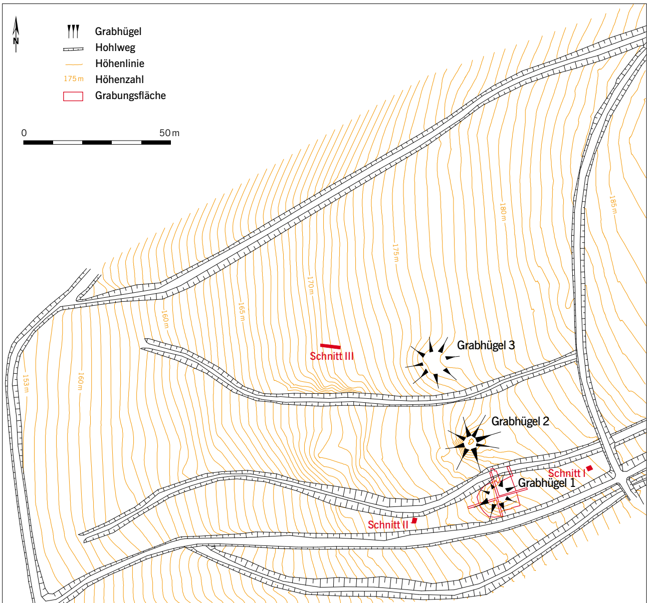
Abb. 3 Vermessungsplan des Geländes am Eichberg im Umfeld des untersuchten Grabhügels 1. Zwischen den Grabhügeln verlaufen alte, nicht mehr genutzte Hohlwege. Der Weg südlich des untersuchten Hügels wird heute noch genutzt.
